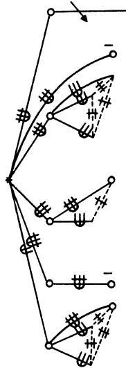
Fig. 13 - Nombre cardinal 2.
