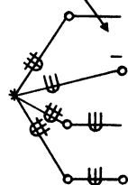
Fig. 9 - Notion d'individu.
