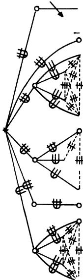
Fig. 14 - Nombre cardinal 3.
