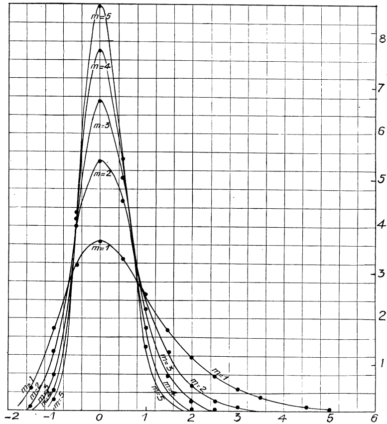
Les distributions finales des m^{\text{ième}} valeurs extrêmes.
