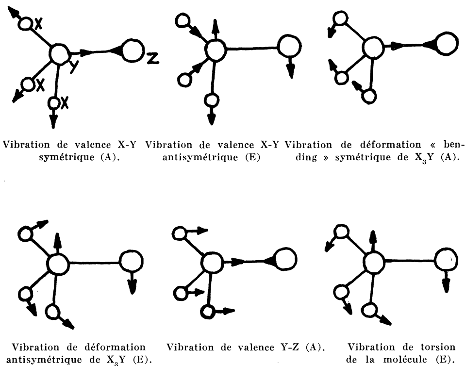
FIG. 2. — Modes de vibration d'une molécule de type H_3N \rightarrow O ou X_3YZ .
