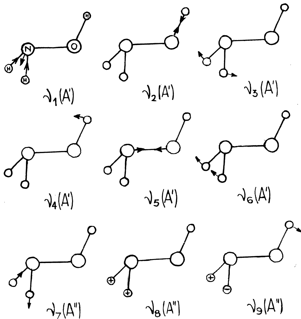
FIG. 1. — Modes de vibration de \text{NH}_2\text{OH} .
