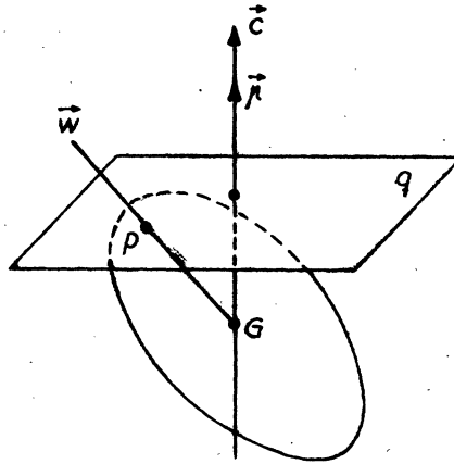
FIG. 4. — Un corps soumis à l'action d'un couple \vec{p} dirigé selon le moment initial \vec{c}_0 se meut d'accord avec la règle de POINSON.
