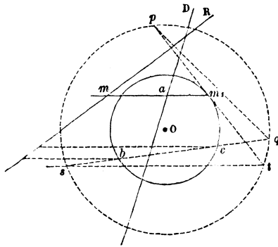
Ombre portée par le conoïde sur lui-même. — Projection verticale.
