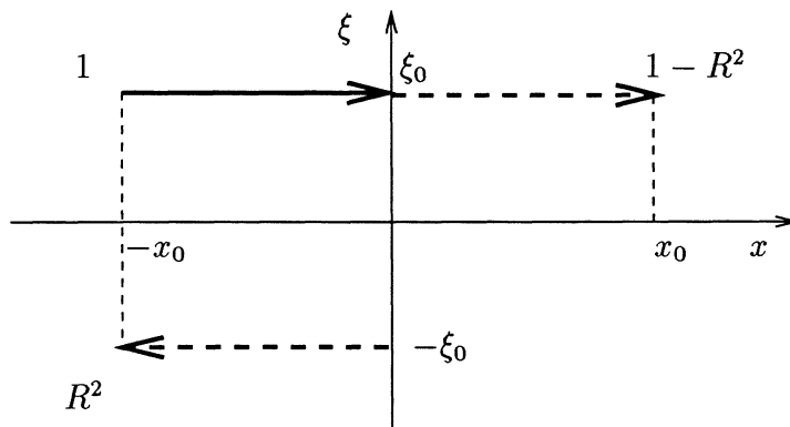
Evolution de la mesure semi-classique \mu(t)
