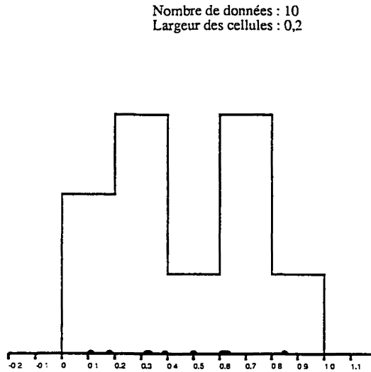
Figure 2. Un histogramme.
