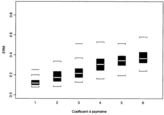
(b) Estimateur 1, \alpha = 95\%
