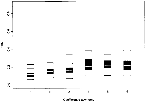
(d) Estimateur 2, \alpha = 95\%
