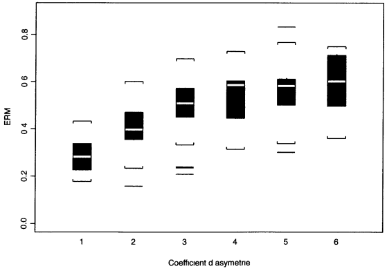
(c) Estimateur 2, \alpha = 5\%
