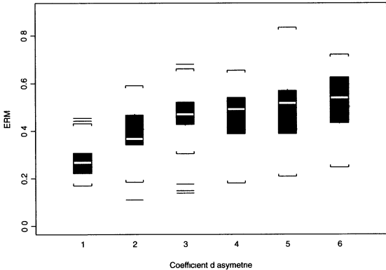
(e) Estimateur 3, \alpha = 5\%
