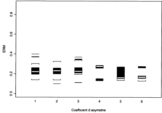
(a) Estimateur 1, \alpha = 5\%
