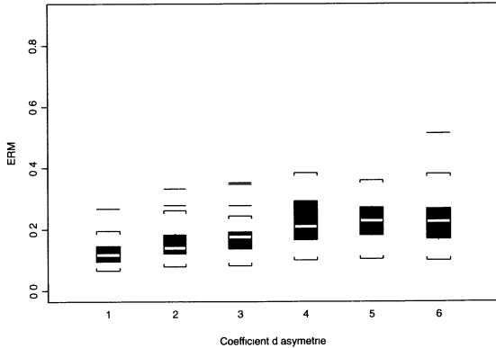
(f) Estimateur 3, \alpha = 95\%
