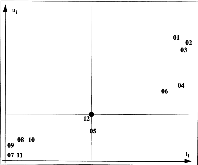
FIGURE 3 Graphique (t_1, u_1)
