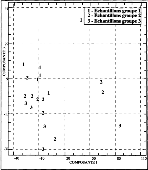
FIGURE 20 Analyse en composantes principales de la matrice X, composantes principales 1 et 3
