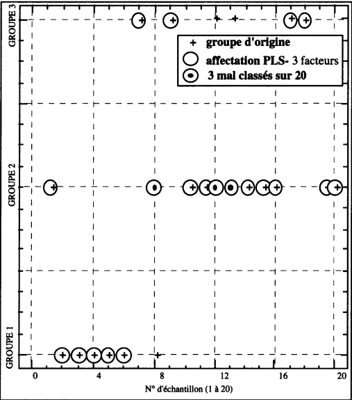
FIGURE 24 Régression PLS de Y sur X
