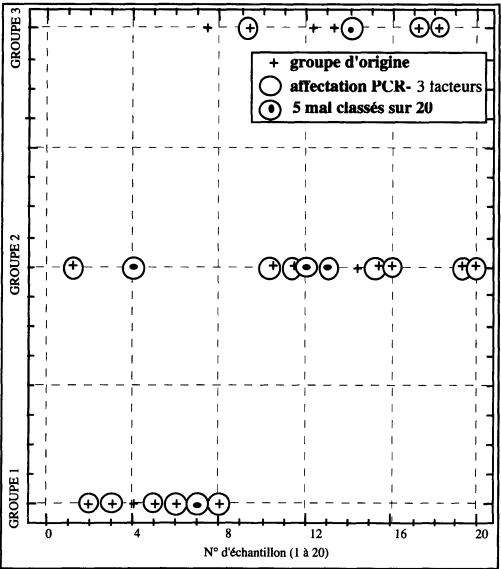
FIGURE 21 Régression sur composantes principales
