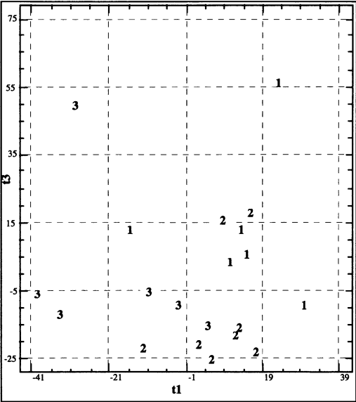
FIGURE 23 Régression PLS de Y sur X. Représentation des échantillons dans le plan t_1, t_3
