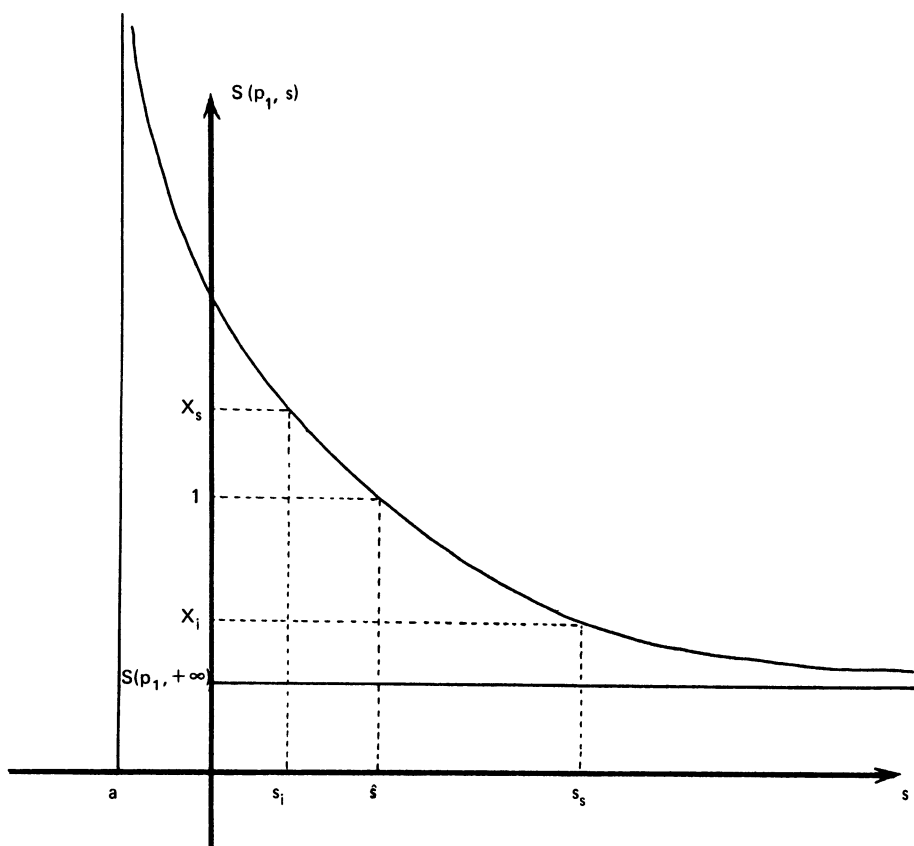
Figure 3. — Représentation graphique de calcul de l'estimation de s et des bornes de l'intervalle de confiance dans le cas où p_1 est supposé connu. Pour des raisons de lisibilité l'échelle des abscisses a été déformée.
