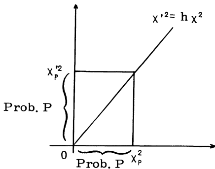
Fig. 2 - Correspondance entre \chi_p^2 et \chi_p'^2 .
