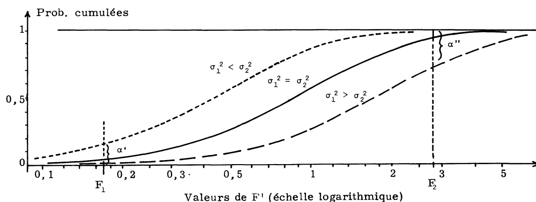
Fig. 8 - Fonction de répartition de F' suivant que \sigma_1^2 est inférieur, égal ou supérieur à \sigma_2^2 . \alpha' , prob. ( 0 < F' < F_1 ) ; \alpha'' , prob. ( F_2 < F' < \infty ). \alpha' = \alpha'' = 0,05 si \sigma_1^2 = \sigma_2^2 .
