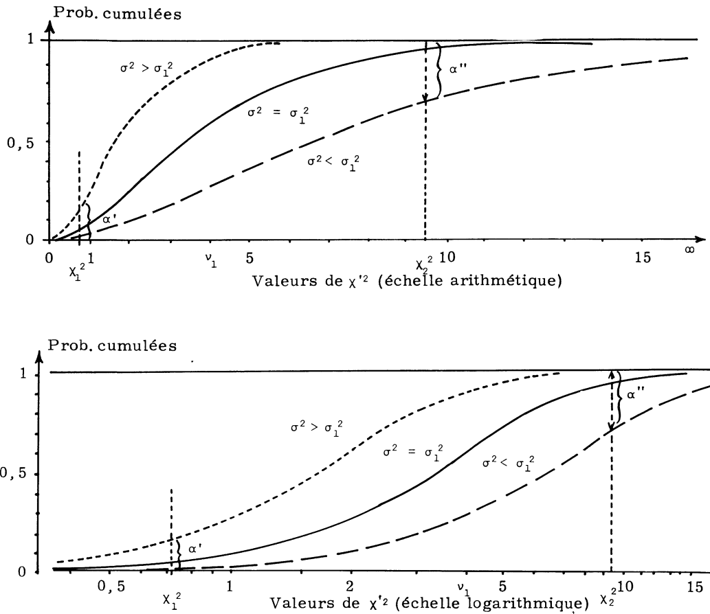
Fig. 3 - Fonction de répartition de \chi'^2 suivant que \sigma^2 est supérieur, égal ou inférieur à \sigma_1^2 . \alpha' , prob. (0 < \chi'^2 < \chi_1^2) ; \alpha'' , prob. (\chi_2^2 < \chi'^2 < \infty) . \alpha' = \alpha'' = 0,05 si \sigma^2 = \sigma_1^2 .
