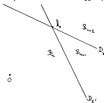
Fig. 4 : point triple
