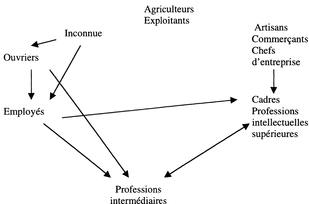
Figure 1 : Graphe des écarts à l'indépendance positifs pour le Tableau 1 (d'après Gollac, Laulhé, Soleilhavoup, 1988)
