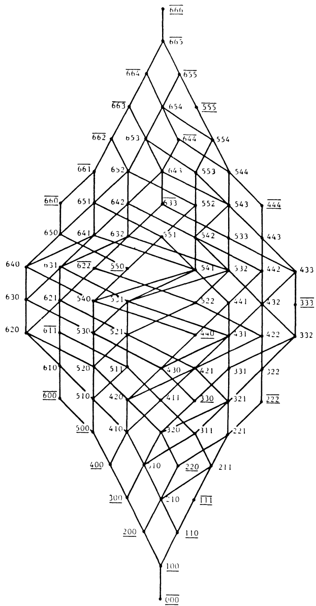
Figure 2. : Le treillis distributif des 84 patrons saturés. (on a représenté deux des figurations possibles de ce treillis)
