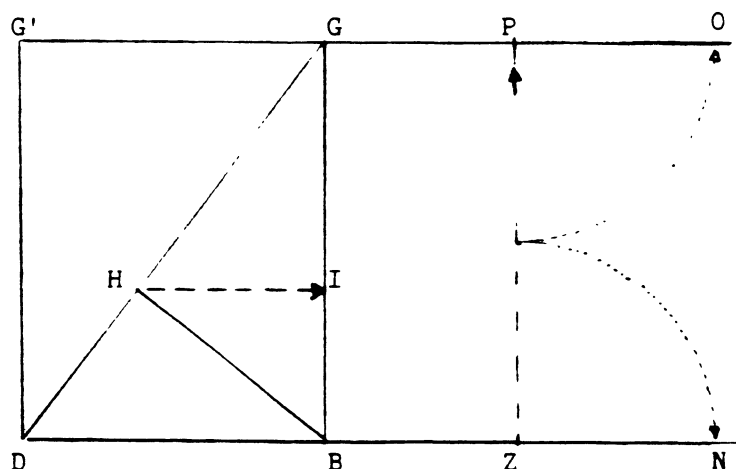
Figure 6 : Le rectangle \sqrt{\varnothing}
