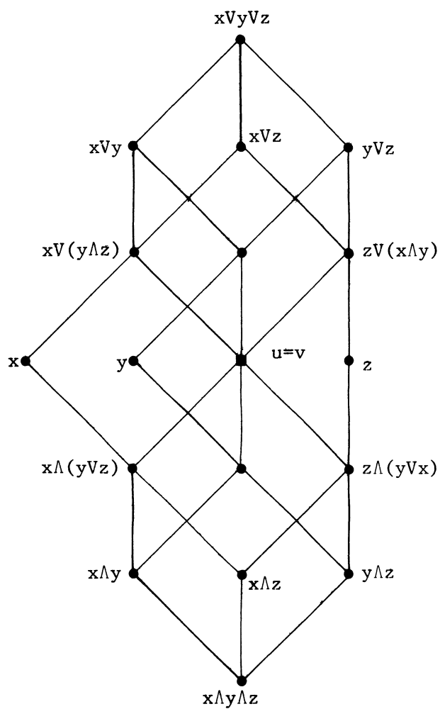
Fig.1. Triplet distributif et sa médiane
