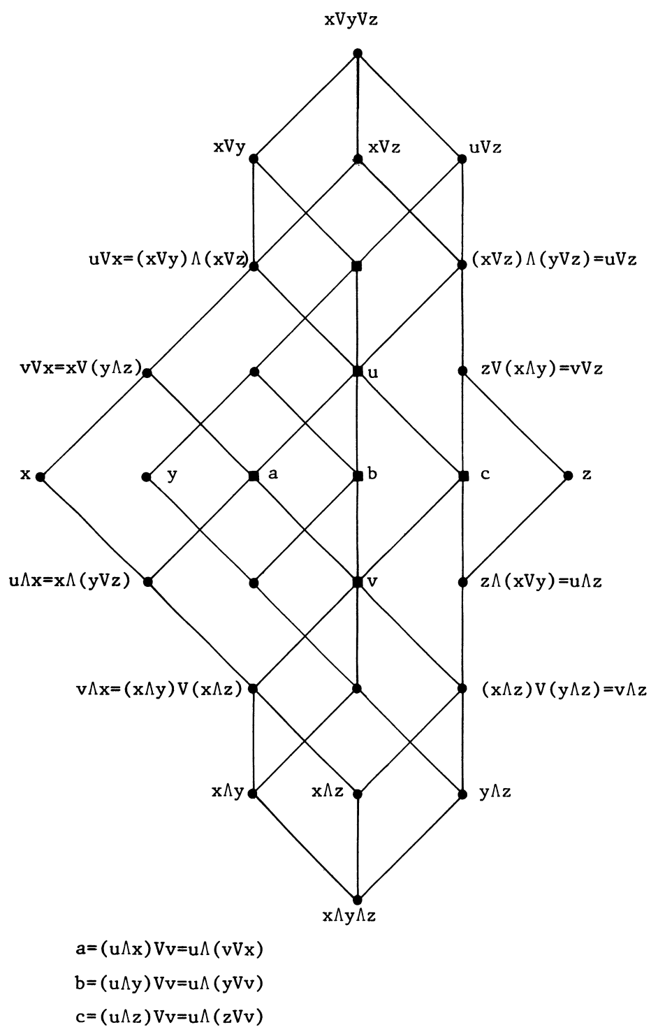
Fig.3. Treillis modulaire engendré par un triplet (x, y, z) et l'intervalle médian [u, v]
