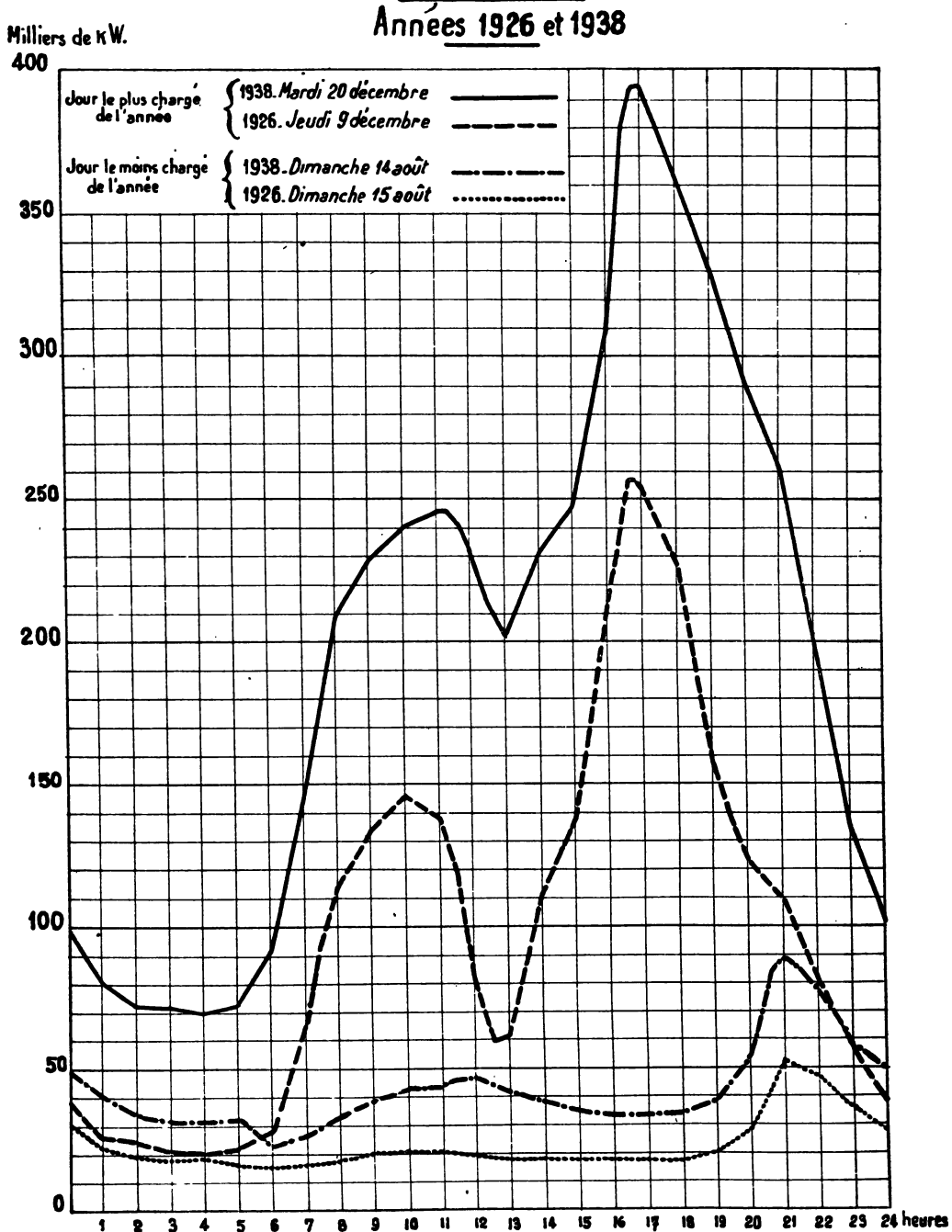
Figure 1 Puissances instantanées à Paris, le jour le plus chargé et le jour le moins chargé de l'année
