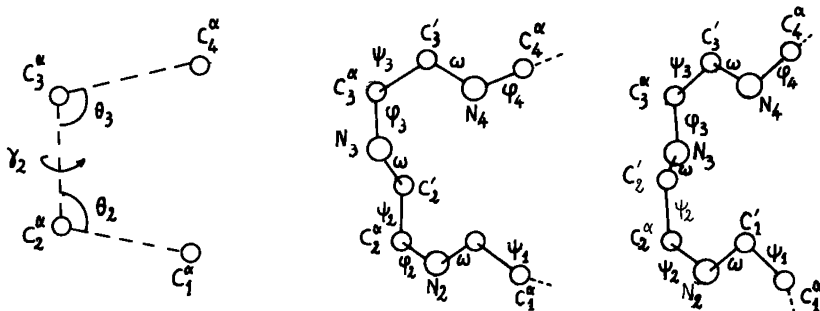
Figure 3 : à droite, deux modèles (I et II) de tournant \beta dans la chaîne d'un polypeptide, réalisés par le jeu d'angles de torsion différents ; à gauche schéma de la chaîne des carbones \alpha .
