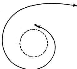
(b) h^2 > 27 .
