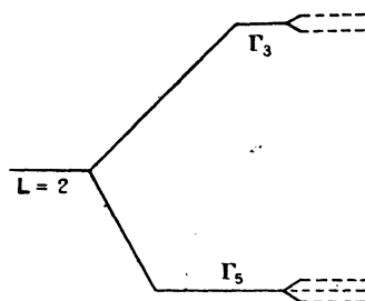
Fig. 10. — Dédoublé d'un état D dans un champ cubique. Les lignes en pointillé représentent la décomposition additionnelle dans le cas d'une symétrie moindre. La figure 10 s'applique à un électron individuel, au lieu d'un atome dans un état collectif D, si le champ cristallin est suffisamment fort pour que le nombre quantique L perde sa signification.
