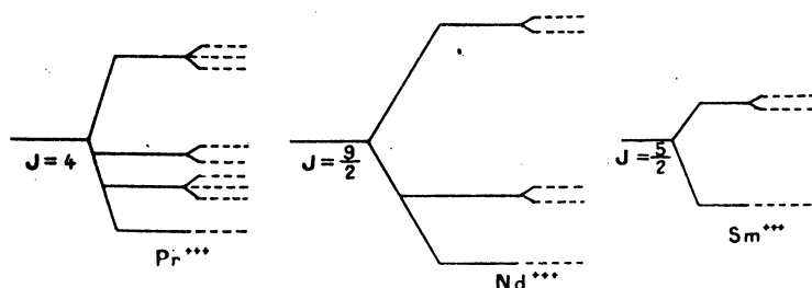
Fig. 7. — Dédoubllement des composantes les plus basses des multiplets du Pr, Nd et Sm dans un champ cubique. Les lignes en pointillé donnent la décomposition additionnelle si le champ n'est pas cubique, et n'a, par exemple, qu'une symétrie rhombique ou trigonale. En tout cas les niveaux de Nd +++ et Sm +++ restent doublement dégénérés, c'est-à-dire, chaque ligne pointillée du Nd +++ ou Sm +++ représente deux niveaux.
