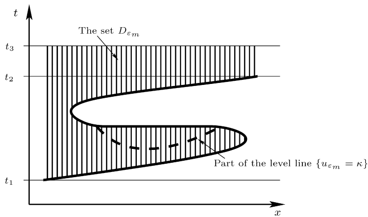
Fig. 5. The set D_{\epsilon_m} .
