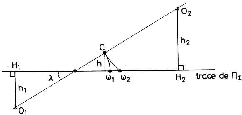
FIG. 1. — Dans le plan vertical passant par O_1 et O_2 , centre des sphères de rayon R tangentes en C. Dans la limite h \rightarrow 0 , \Delta \equiv \omega_1\omega_2 \simeq h^2/R \cos^3 \lambda où \lambda est l'angle de O_1O_2 avec le plan de section, de trace H_1H_2 dans le plan de la figure.
