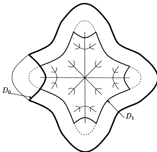
FIG. 2 – Les pièces D_0 et D_1 délimitées par des équipotentielles et des rayons externes.
