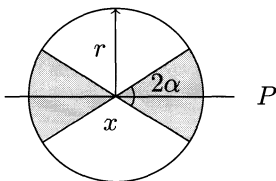
Figure 1. Le cône C(x, r, \varepsilon, P) pour n = 2 et d = 1 ( \varepsilon = \sin \alpha )
