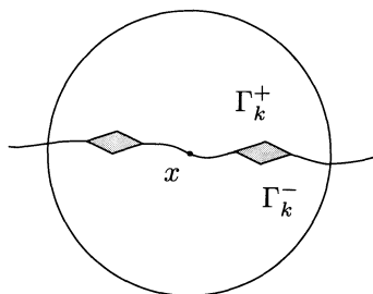
Figure 2. Dans B(x, r_k) , les points de E appartiennent à \Gamma_k^+ \cap \Gamma_k^- ou sont dans les zones hachurées (propriété (119) pour n = 2, d = 1 ). On voit bien alors que, pour t < r_k , \beta_q(x, t, E) est dominé par \beta_q(x, t, \Gamma_k^+ \cup \Gamma_k^-) .
